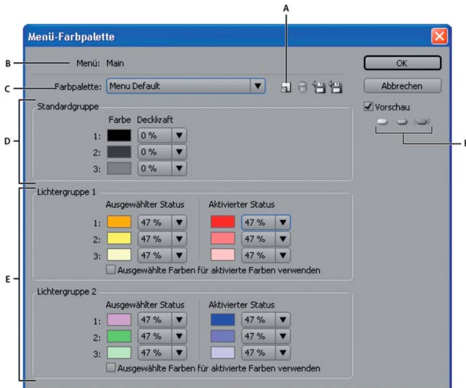
Dialogfeld „Menü-Farbpalette“
