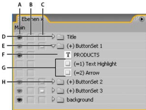
Ebenenfenster
