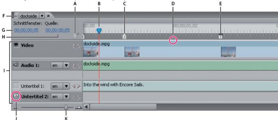
Schnittfenster-Viewer
