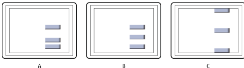
Verteilte Objekte
