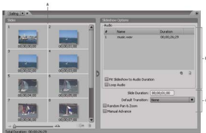
Bildschirmpräsentations-Viewer
