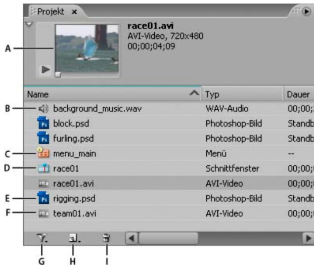
Projektfenster
